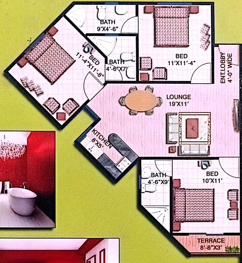
TYPE - C
